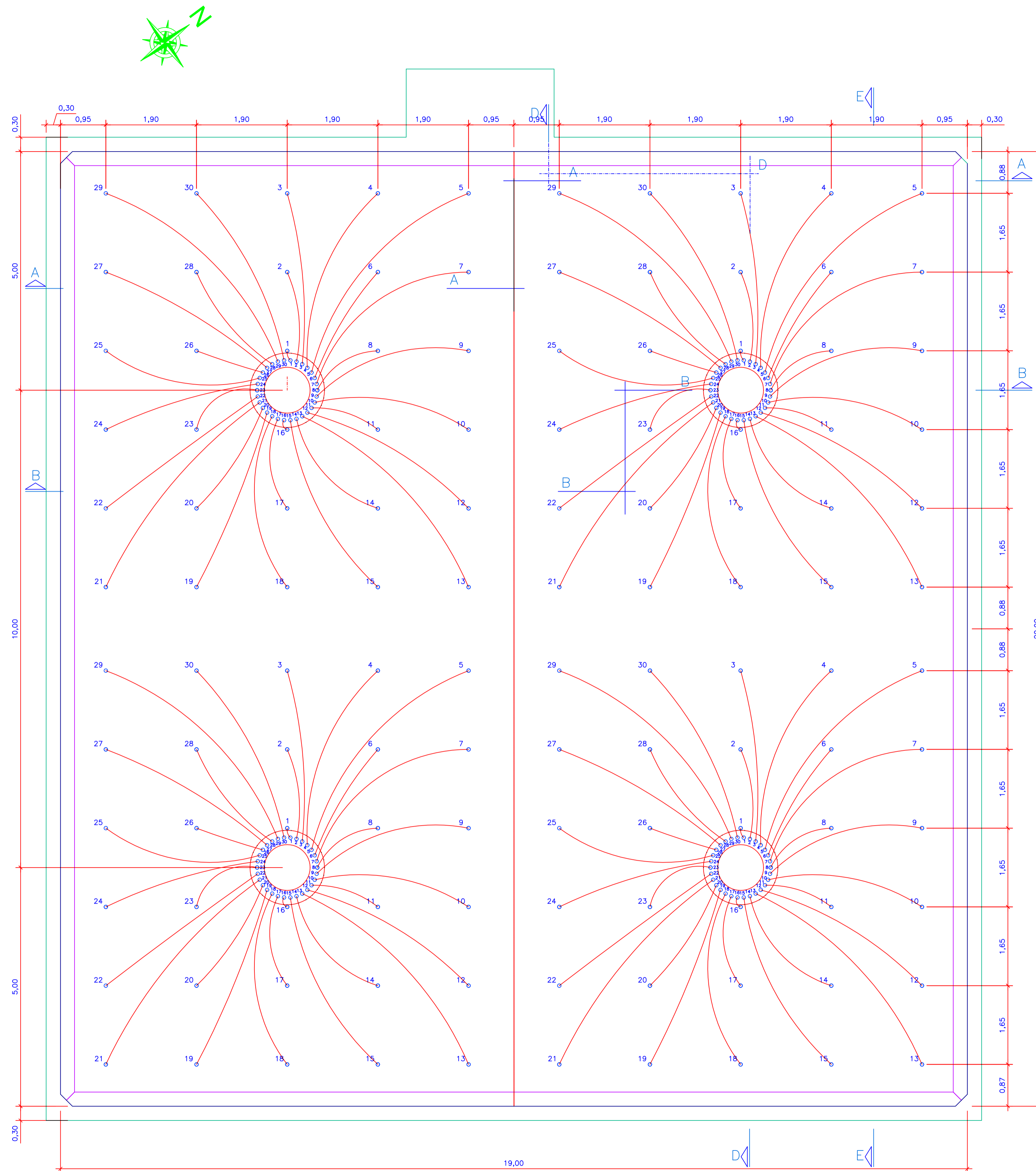
ESQUEMA DE DISTRIBUIÇÃO DOS TUBOS PEAD 75mm NO DIGESTOR ESC: 1:50
