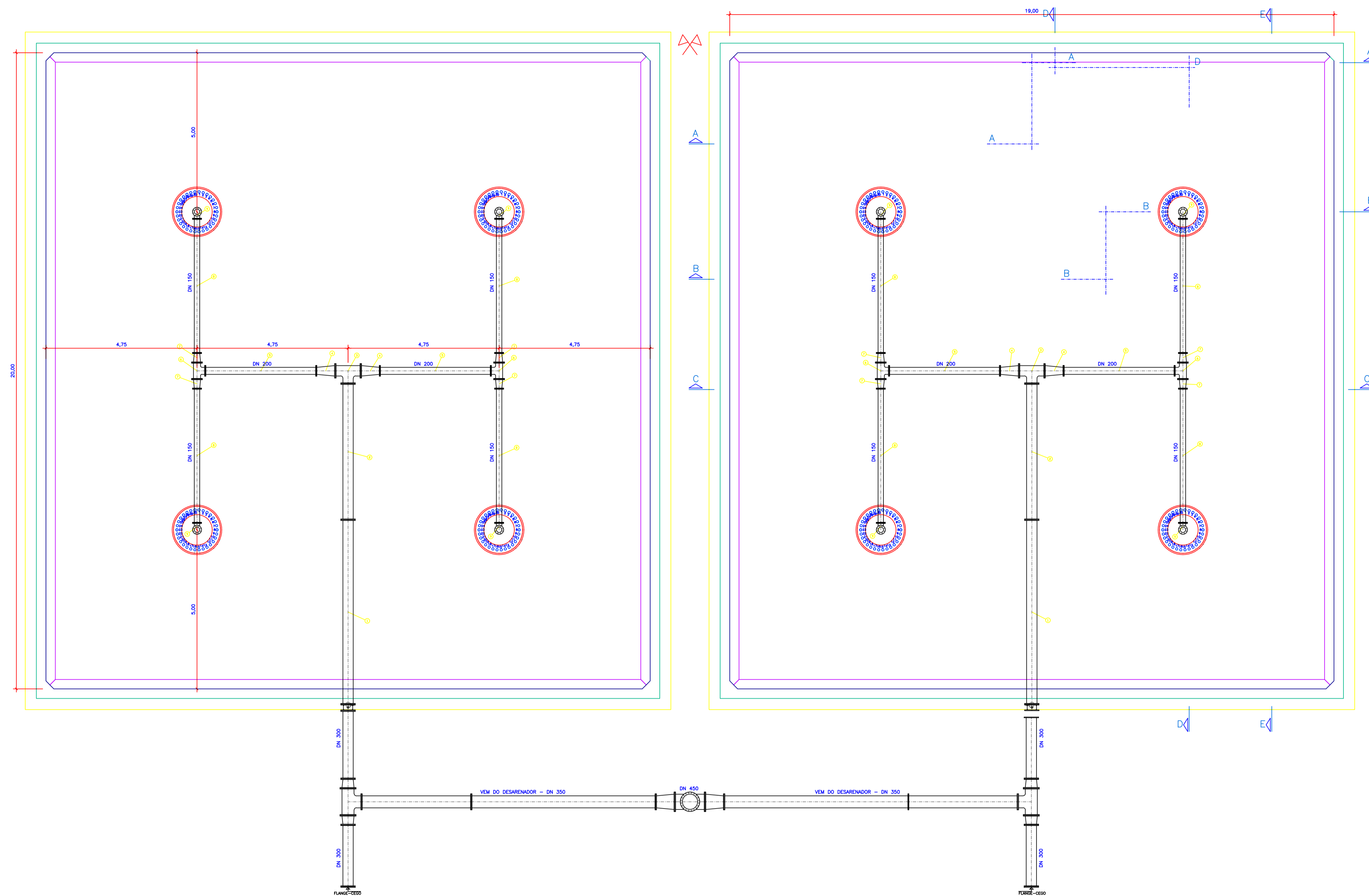
PLANTA TUBOS DE ALIMENTAÇÃO ESC: 1:75
